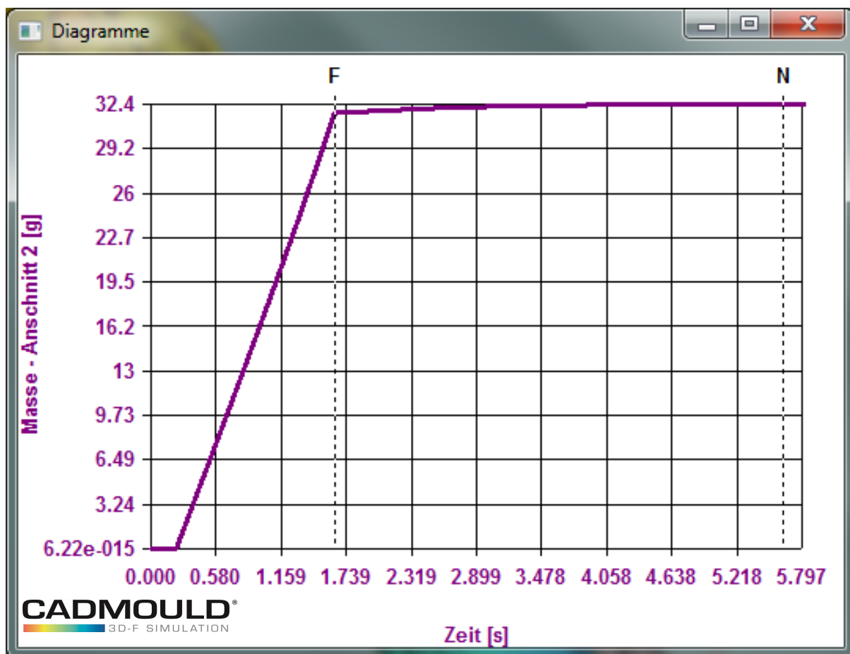
Diagramm - Masse – Anschnitt
